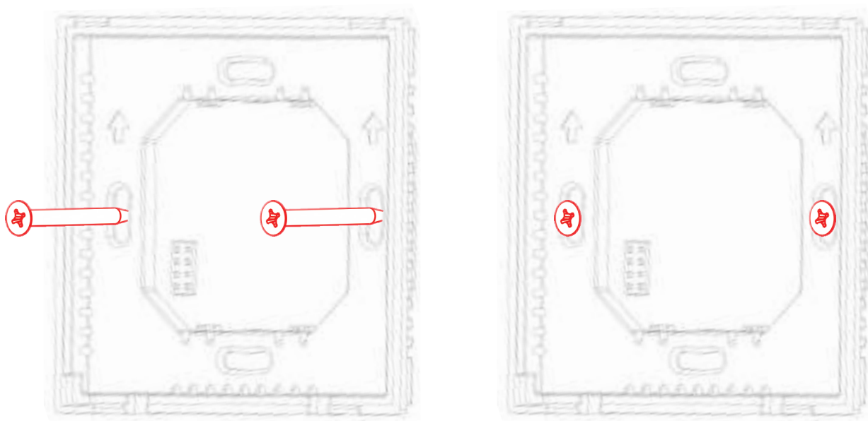
Рис. 5 Схема расположения винтов
