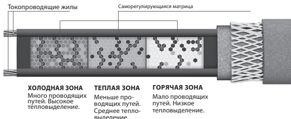
Рисунок 2. Принцип саморегулирования кабеля
