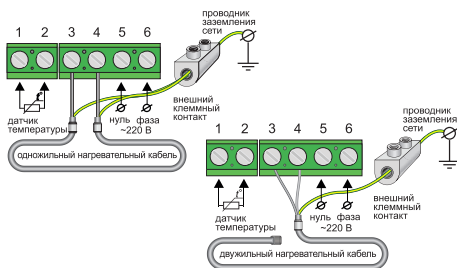
Рис. 6. Схема подключения к 3-х проводной сети питания нагревательных секций и матов
