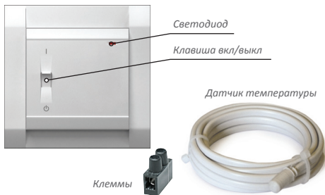
Рис. 3. Исполнительный модуль TP 810
