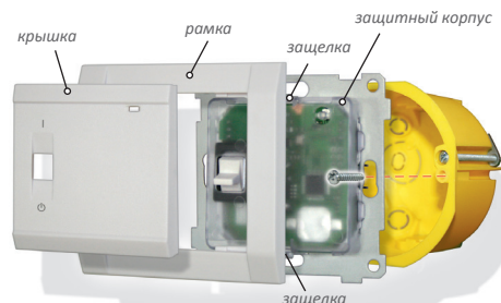
Рис. 7. Снятие крышки прибора
